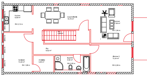
Grundriss Obergeschoss
