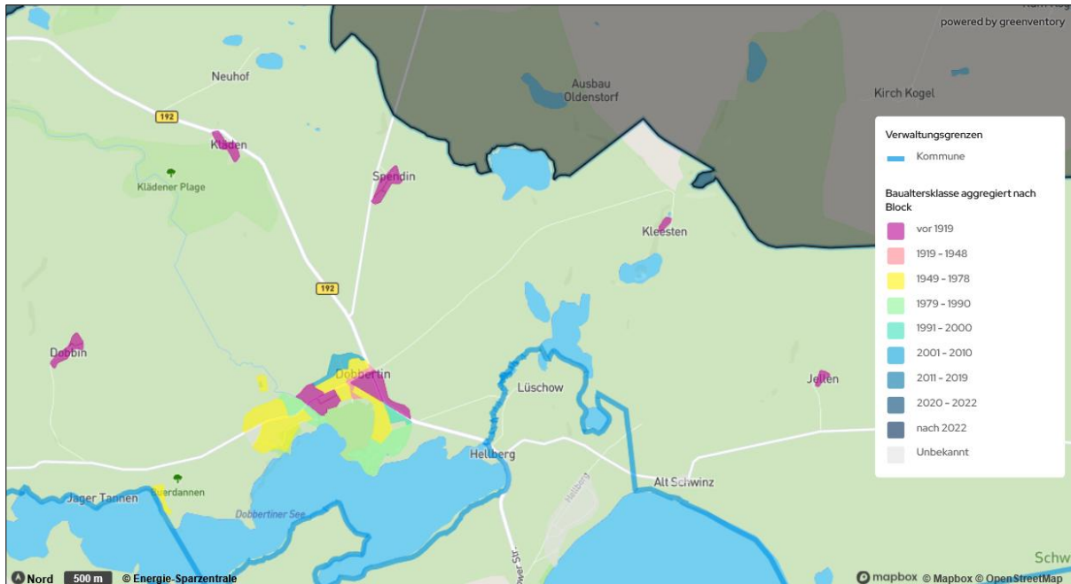
Abbildung 5: Verteilung der Baualtersklassen für Gebäude – Dobbertin
