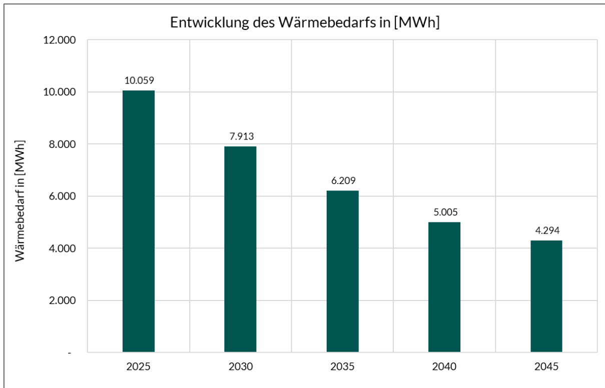
Abbildung 36: Wärmebedarfsentwicklung durch Heizungstausch in WG
