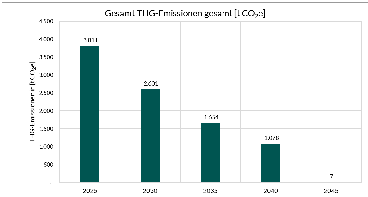
Abbildung 44: Kombination der Teilszenarien der THG-Emissionen im zeitlichen Verlauf
