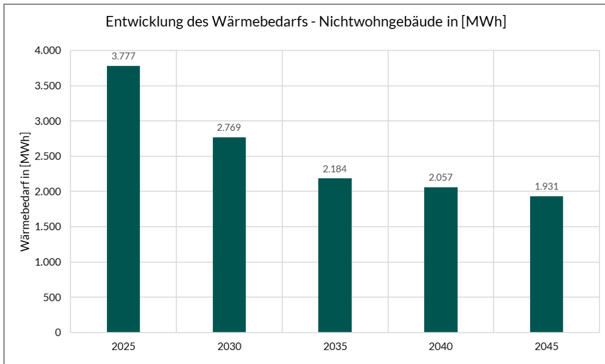
Abbildung 32: Wärmebedarf & Wärmebedarfsreduktion im Ziel- & Zwischenjahr für NWG
