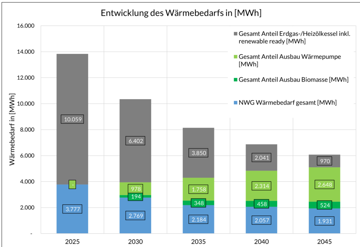
Abbildung 42: Verteilung des Endenergiebedarfs nach Energieträgern im zeitlichen Verlauf
