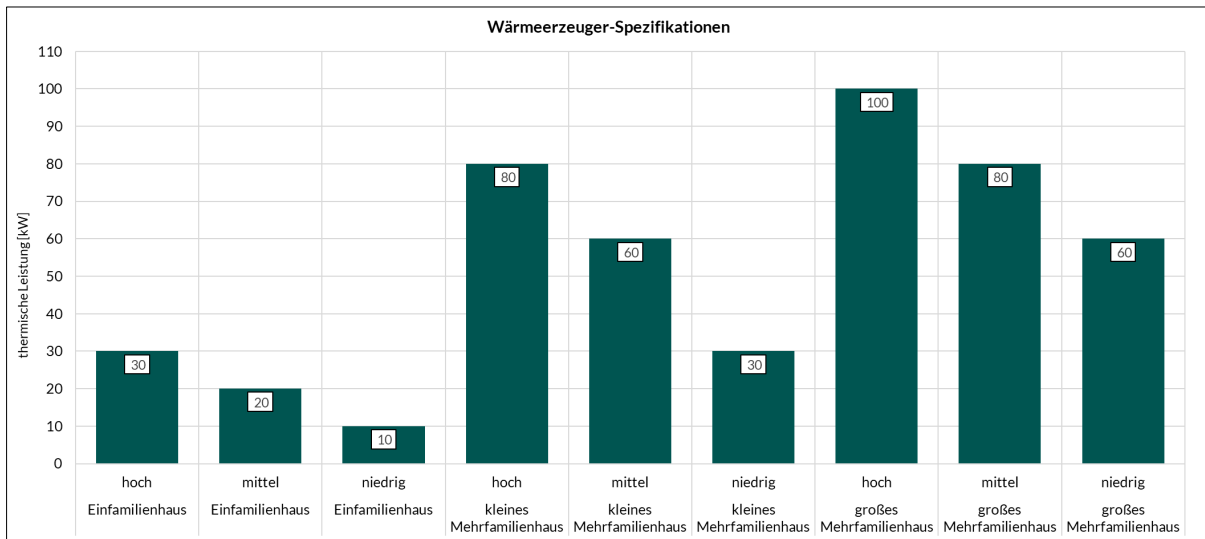
Abbildung 27: Wärmeverkostungen - Wärmeerzeugerspezifikationen (Nennleistung)
