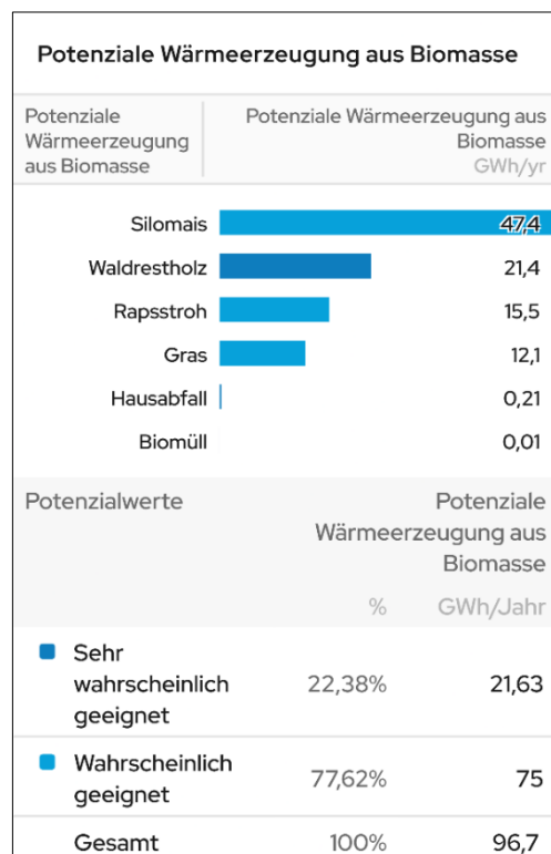
Abbildung 23: Potenziale Wärmeerzeugung aus Biomasse
