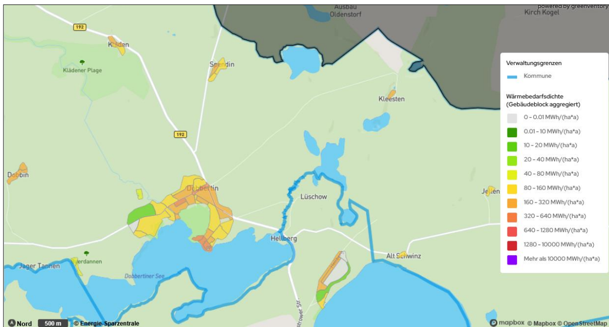
Abbildung 7: Verteilung der Wärmebedarfe je nach Baublock – Dobbartin
