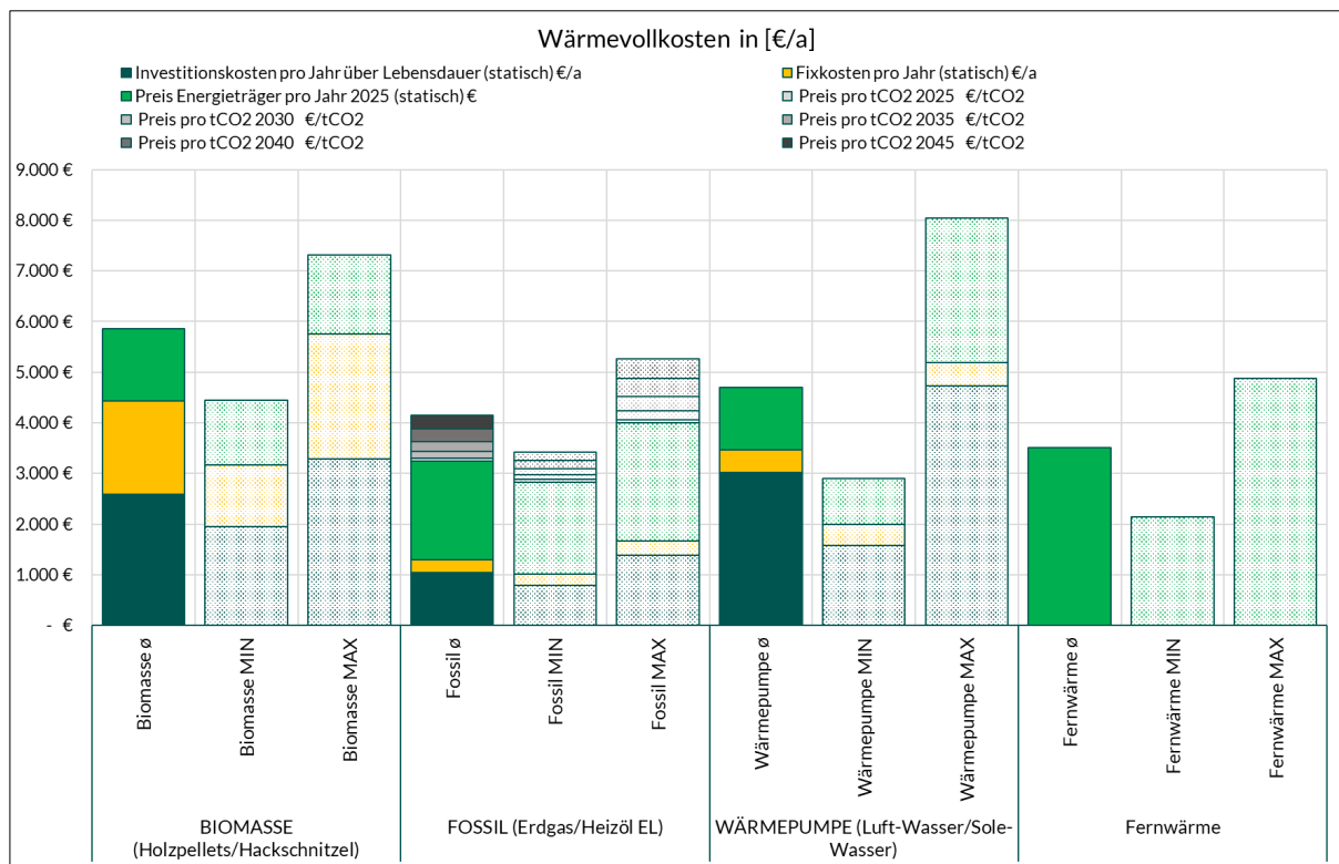
Abbildung 28: Wärmevollkosten – Verteilung Kostenarten (EFH - mittlerer Wärmebedarf)
