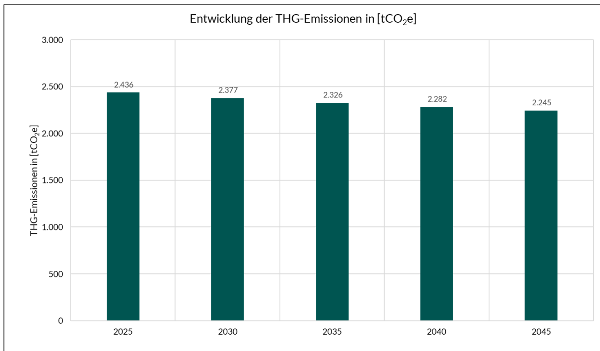
Abbildung 30: THG-Emissionen für eine Sanierungsquote von 0,8 % p. a. für Wohngebäude
