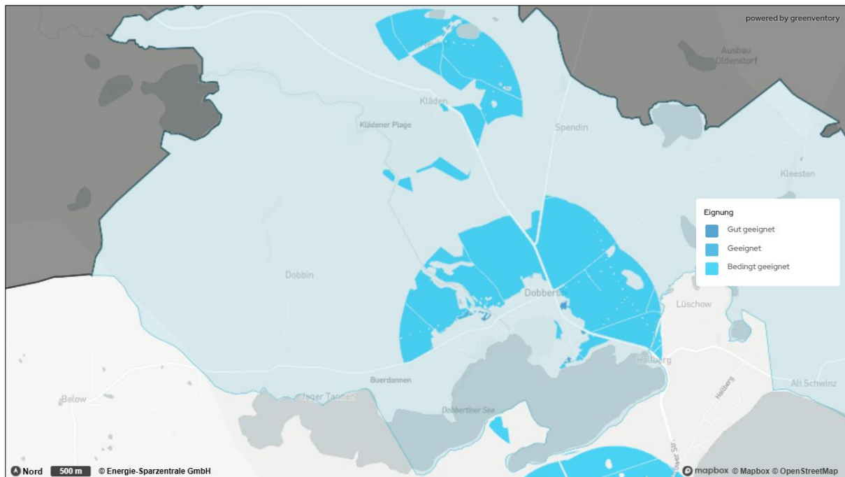
Abbildung 21: Eignungsgebiete Freiflächen-Solarthermie
