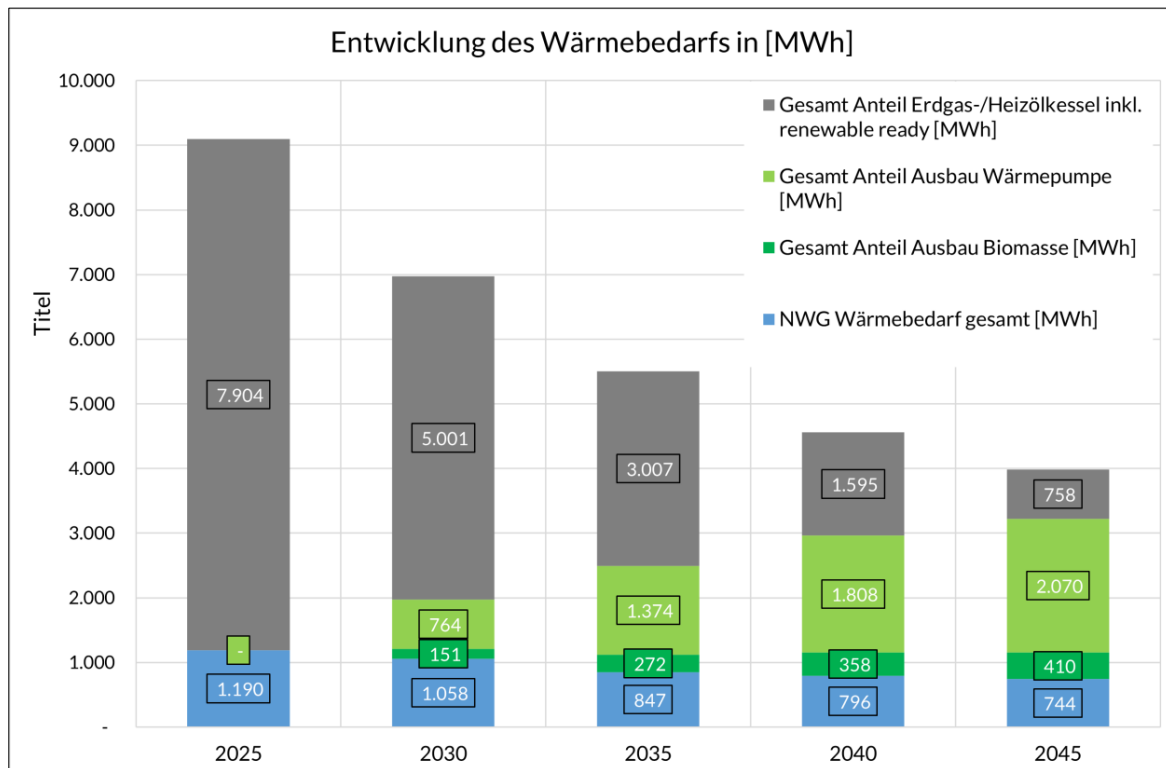
Abbildung 42: Verteilung des Wärmebedarfs nach Energieträgern im zeitlichen Verlauf
