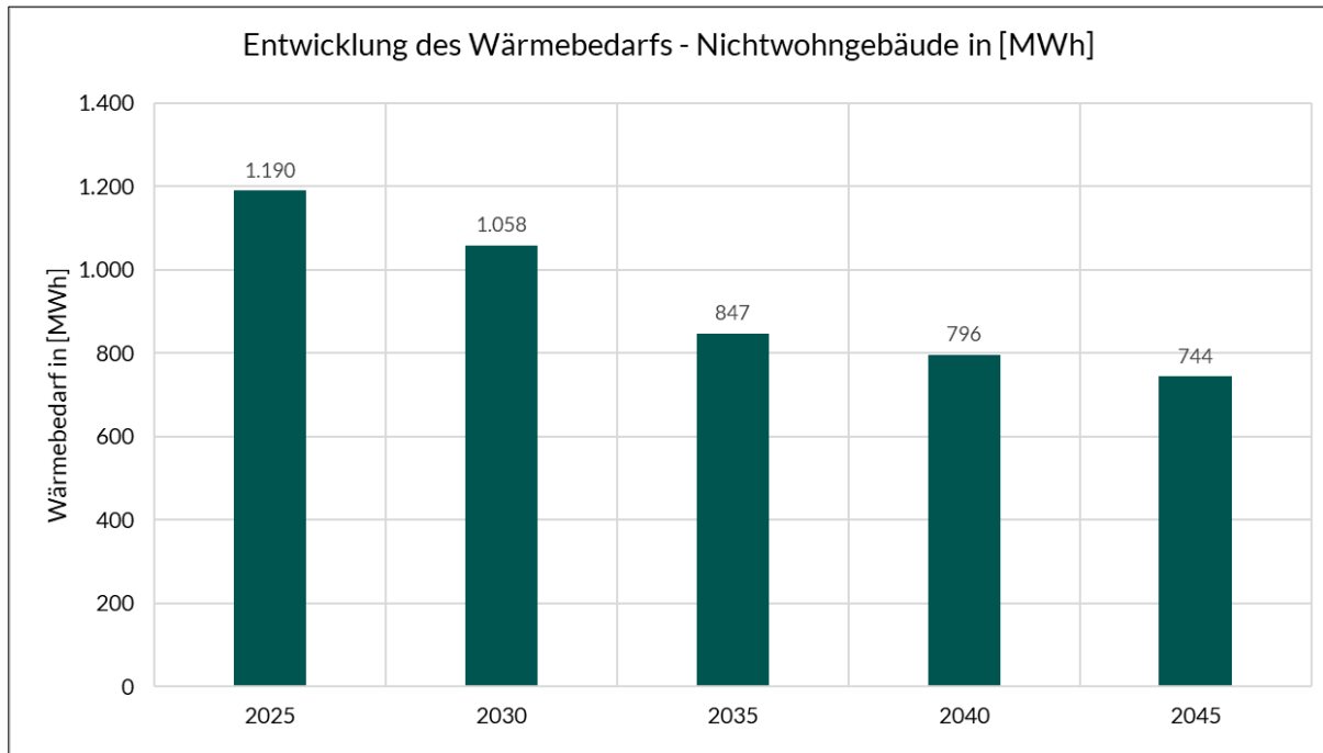
Abbildung 34: Wärmebedarf & Wärmebedarfsreduktion im Ziel- & Zwischenjahr für NWG
