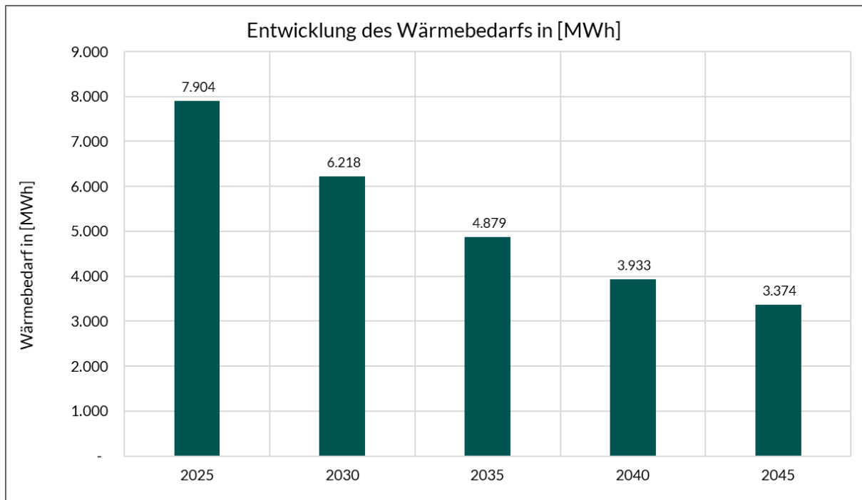
Abbildung 38: Wärmebedarfsentwicklung durch Heizungstausch in WG
