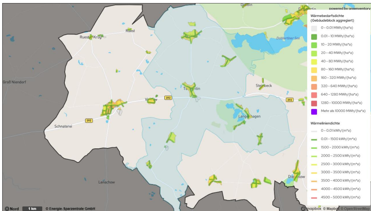
Abbildung 41: Übersicht der geprüften Eignungsgebiete für Wärmenetze - Techentin
