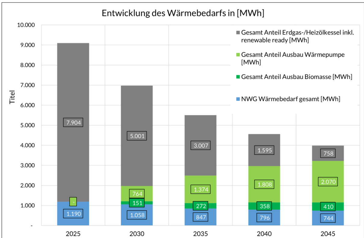
Abbildung 45: Verteilung des Endenergiebedarfs nach Energieträgern im zeitlichen Verlauf
