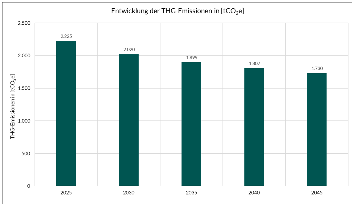
Abbildung 33: THG-Emissionen für eine Sanierungsquote von 2,0 % p. a. für Wohngebäude
