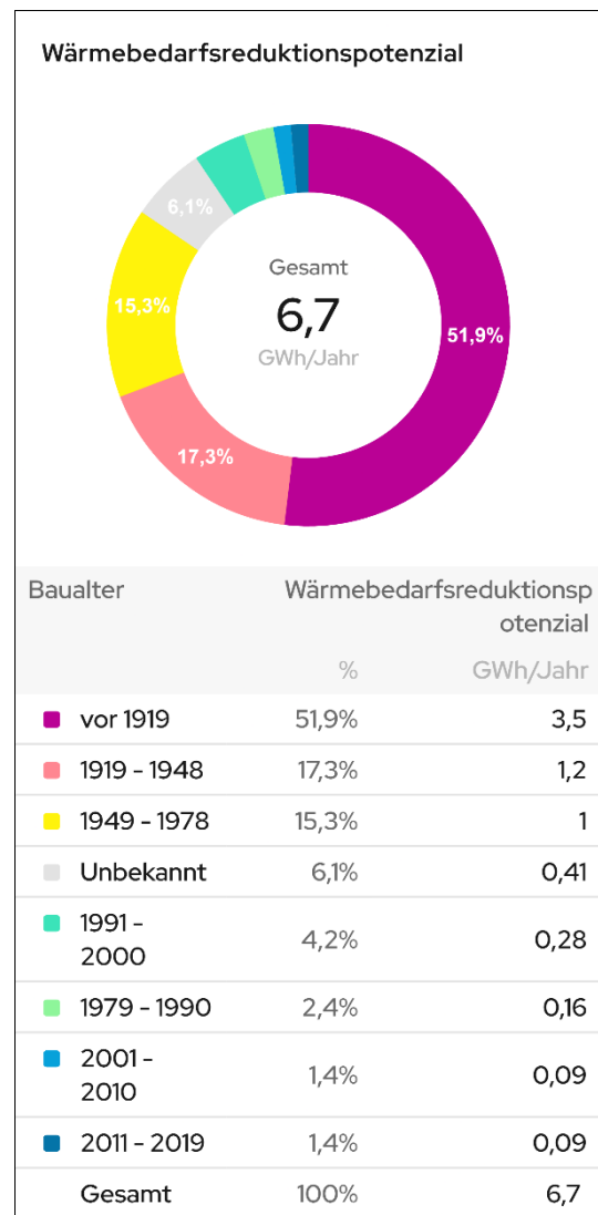
Abbildung 26: Reduktionspotenzial nach Baualterklassen - Techentin
