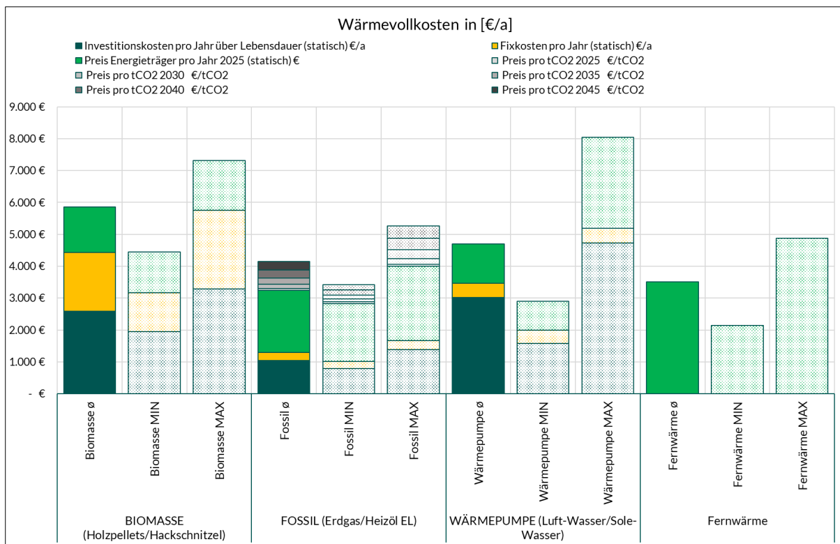
Abbildung 30: Wärmevollkosten - Verteilung Kostenarten (EFH - mittlerer Wärmebedarf)
