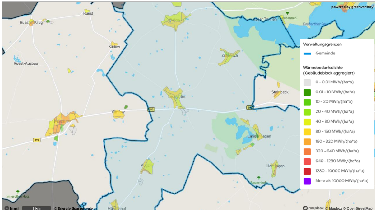
Abbildung 7: Verteilung der Wärmebedarfe je nach Baublock – Techentin
