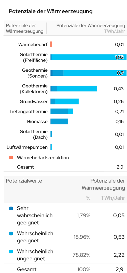
Abbildung 22: Erneuerbare Wärmepotenziale – Techentin
