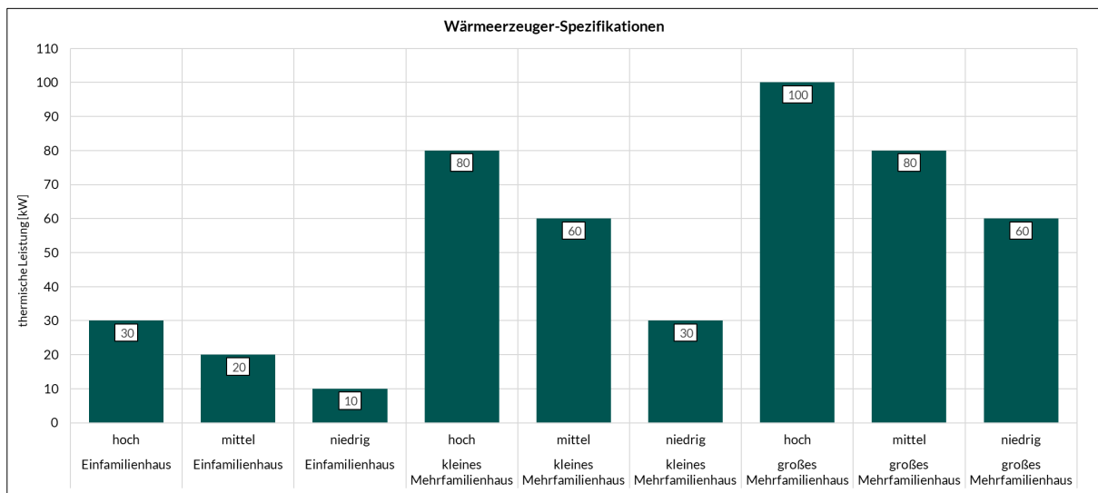
Abbildung 29: Wärmevervollkosten - Wärmeerzeugerspezifikationen (Nennleistung)
