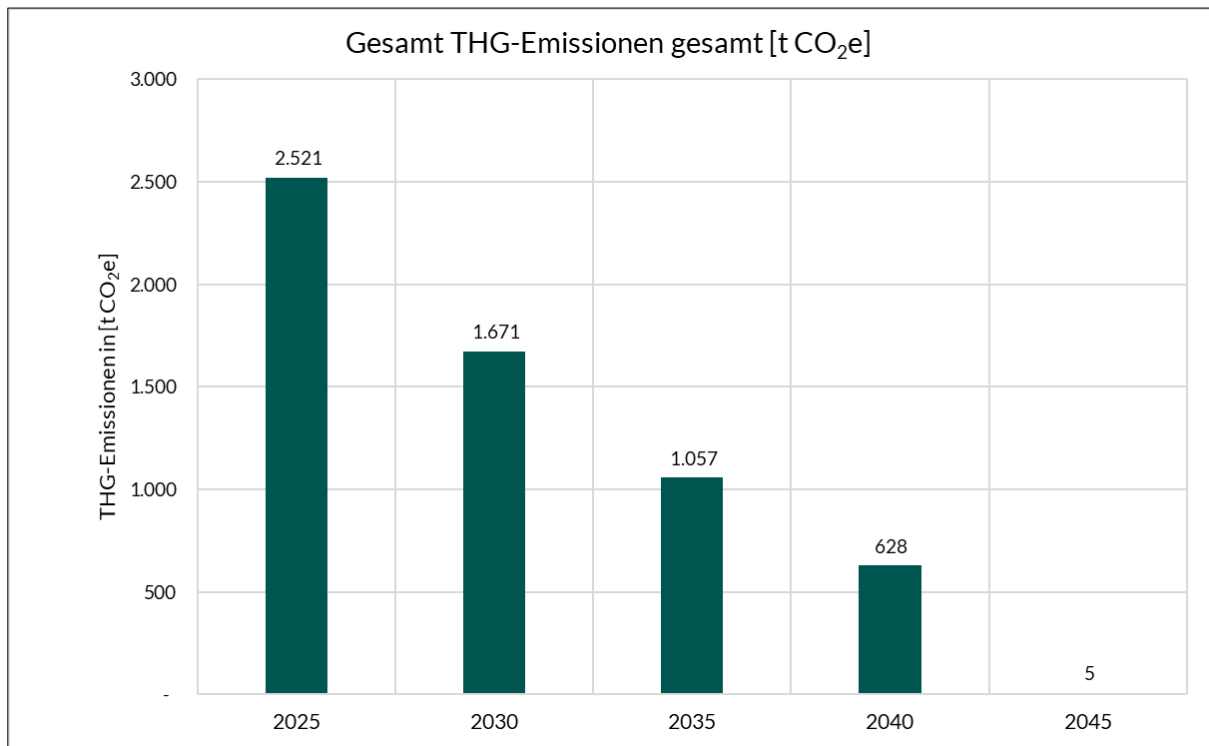
Abbildung 47: Kombination der Teilszenarien der THG-Emissionen im zeitlichen Verlauf
