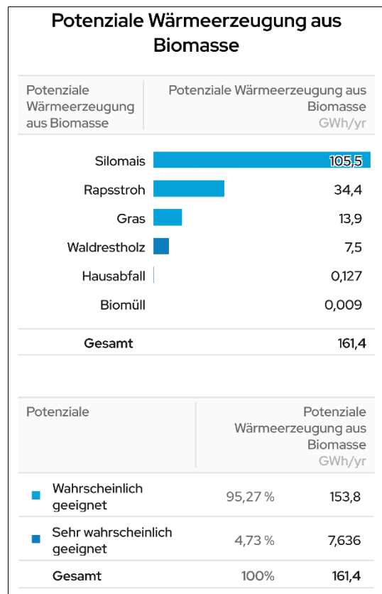
Abbildung 25: Potenziale Wärmeerzeugung aus Biomasse
