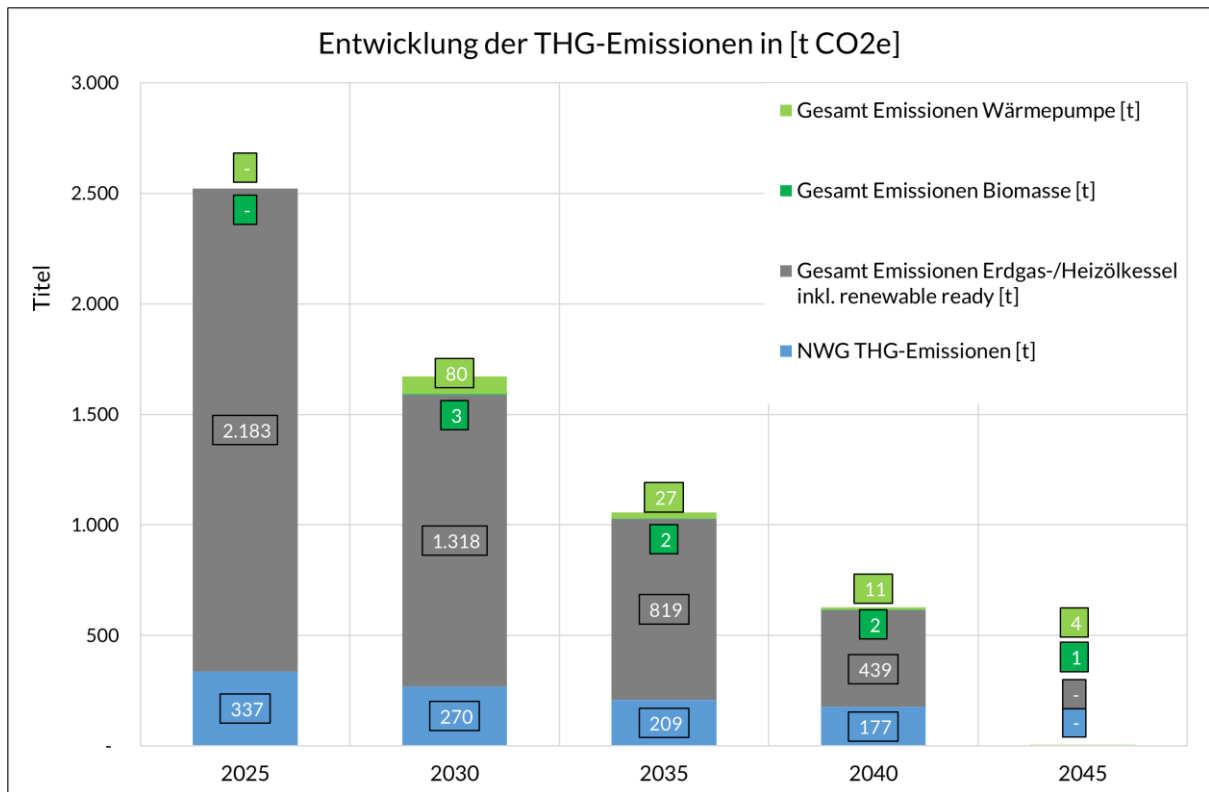
Abbildung 43: Verteilung der THG-Emissionen nach Energieträgern im zeitlichen Verlauf
