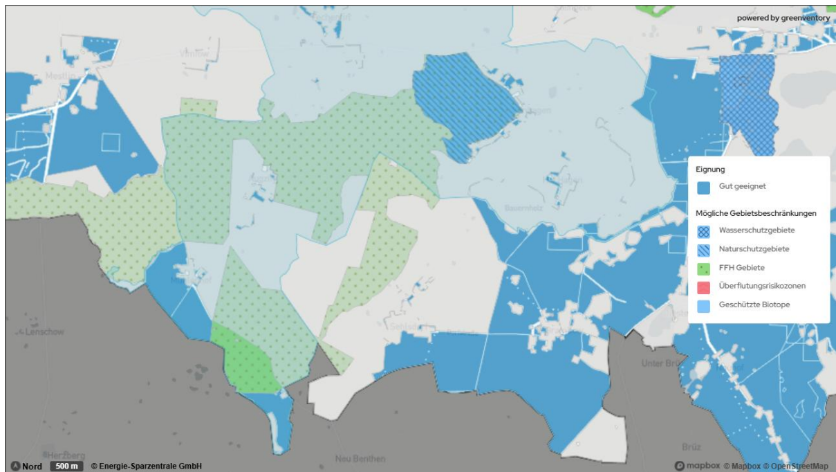
Abbildung 20: Eignungsgebiete Freiflächen-Photovoltaik südlicher Teil von Techentin
